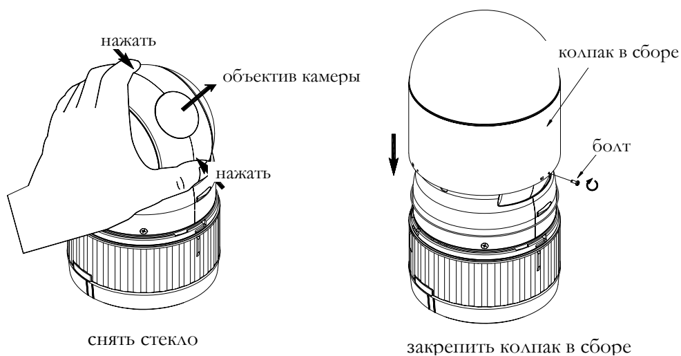
Рис. 2 – Закрепление колпака
