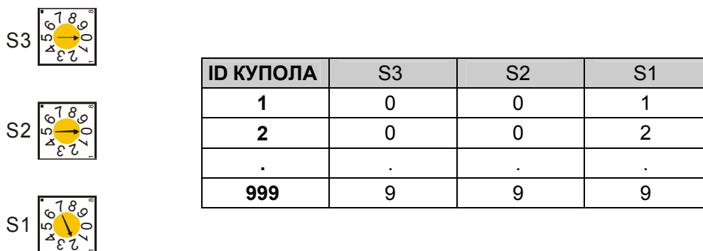
Рис. 8 – Настройка адреса (ID) купольной камеры
