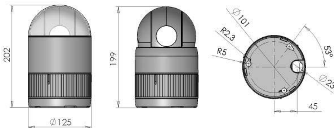
Рис. 10 – Размеры
